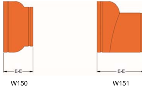
W150
